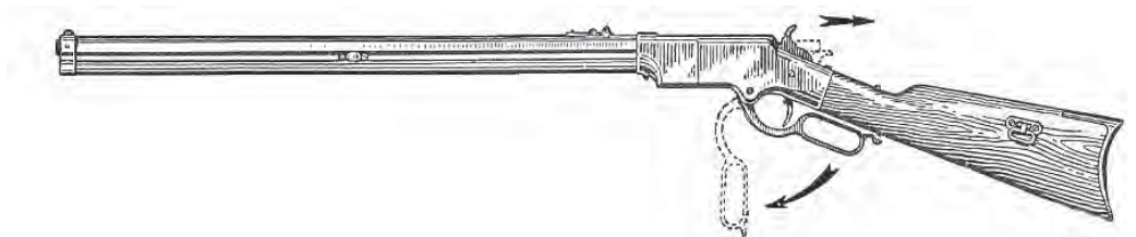
Մենի-Մարտինի 1860թ. օրինակի հրացանները «մրցունակ» էին Բերդանի հրացանների դեմ։ Ղեկավարվող լծակով երկայնակի-սահող փակադակի օգնությամբ կրակված պարկուճը դուրս էր նետվում, իսկ փողատակի պահեստատուփից վերալիցքավորումը կատարվում էր շատ արագ։
