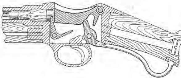
Բ. Փակադակը փակ է
